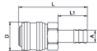
Schlauchtülle
