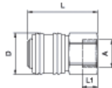
Innengewinde
