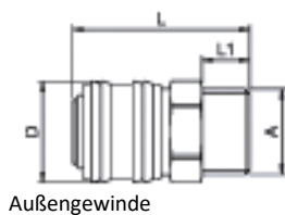
Außengewinde
